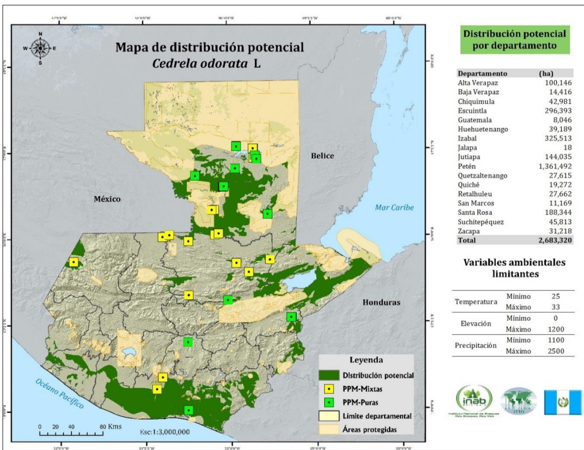
Figura 7. Mapa de distribución potencial de Cedrela odorata L. en el territorio de Guatemala (fuente: Departamento de Investigación Forestal del INAB, 2016).
